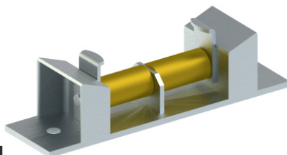
Typ 118 GFH Rollenlager mit seitlicher Führung und Abhebesicherung nur in Kombination mit Gleitunterstützung Typ 180 HS / Katalogseite 120 sowie Typ 171-..HS/Katalogseite 159 +160 verwendbar.
