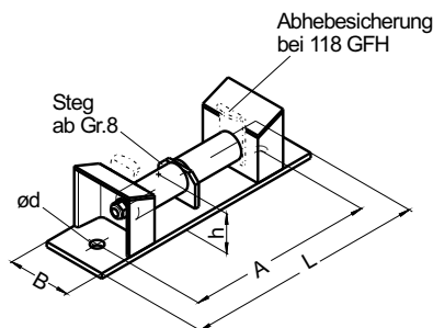
Typ 118 GFH Rollenlager mit seitlicher Führung und Abhebesicherung nur in Kombination mit Gleitunterstützung Typ 180 HS / Katalogseite 120 sowie Typ 171-..HS/Katalogseite 159 +160 verwendbar.
