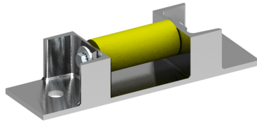
Typ 118 GOF Rollenlager ohne seitlicher Führung
